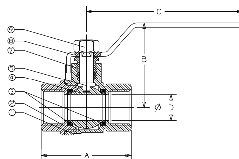
T-FP-40-BSPP BSPP
